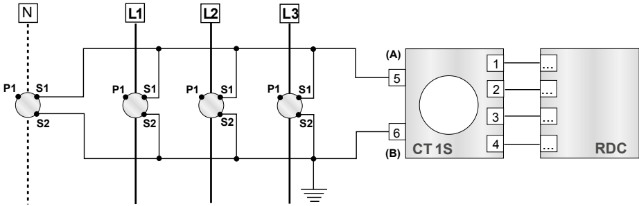
4x Transformadores de medida Serie BH-0.66 (relación In/5) Comprobar sección del transformador
